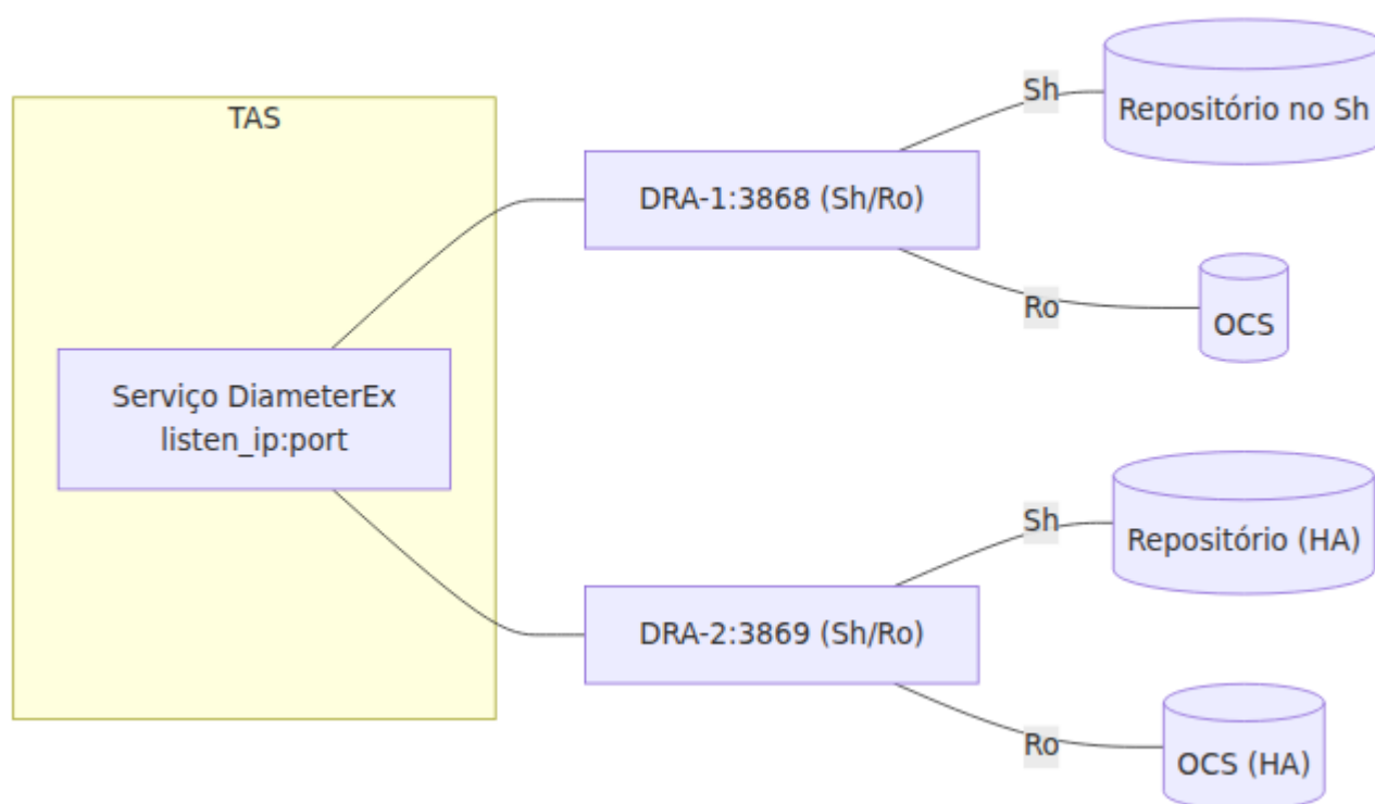
Conectividade do Par Diameter
